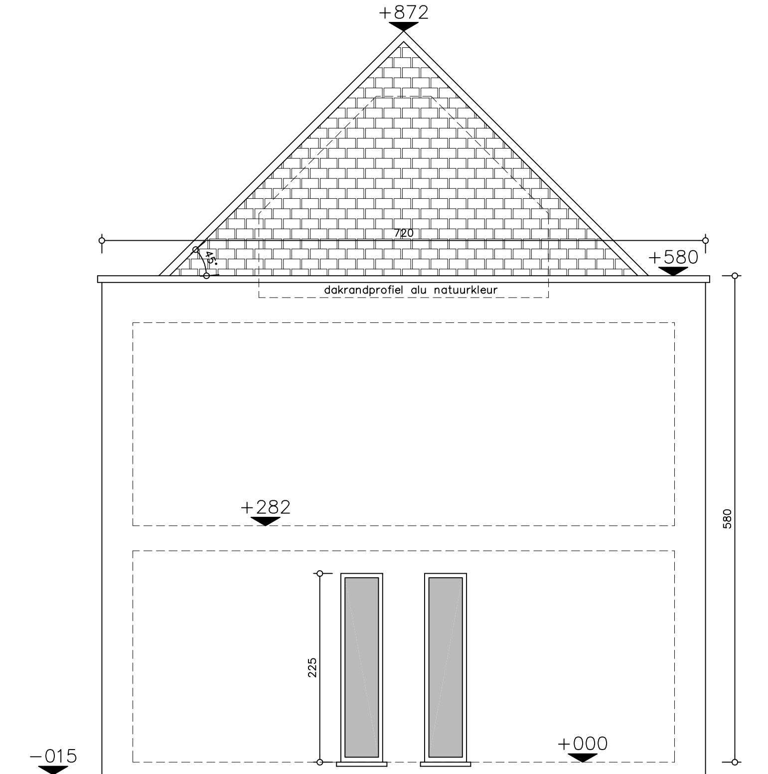
Zijgevel links
