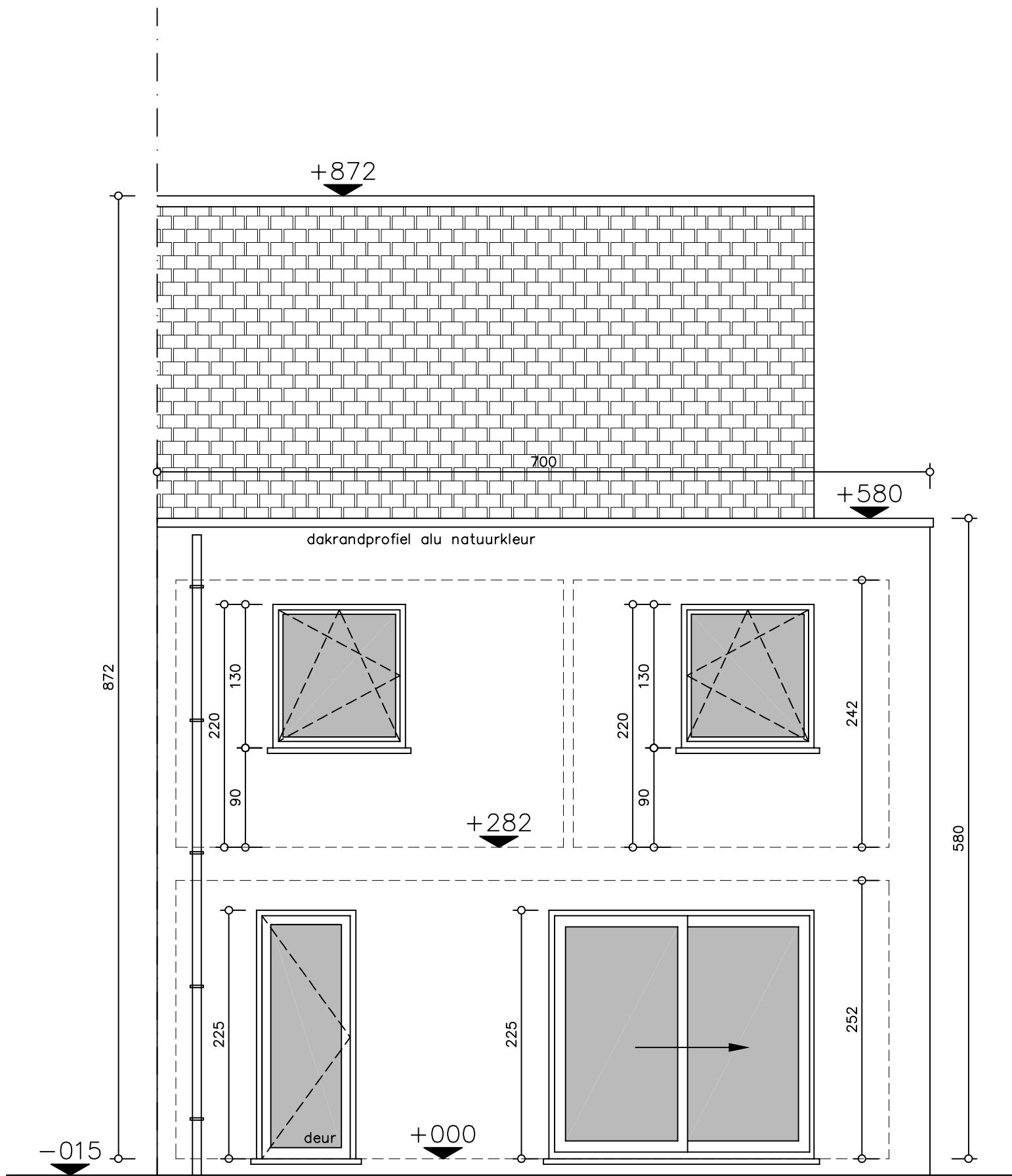
Achtergevel
