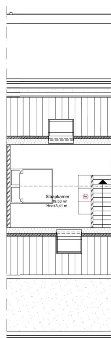
2. Lot 2 - 2e verdieping 1:100
