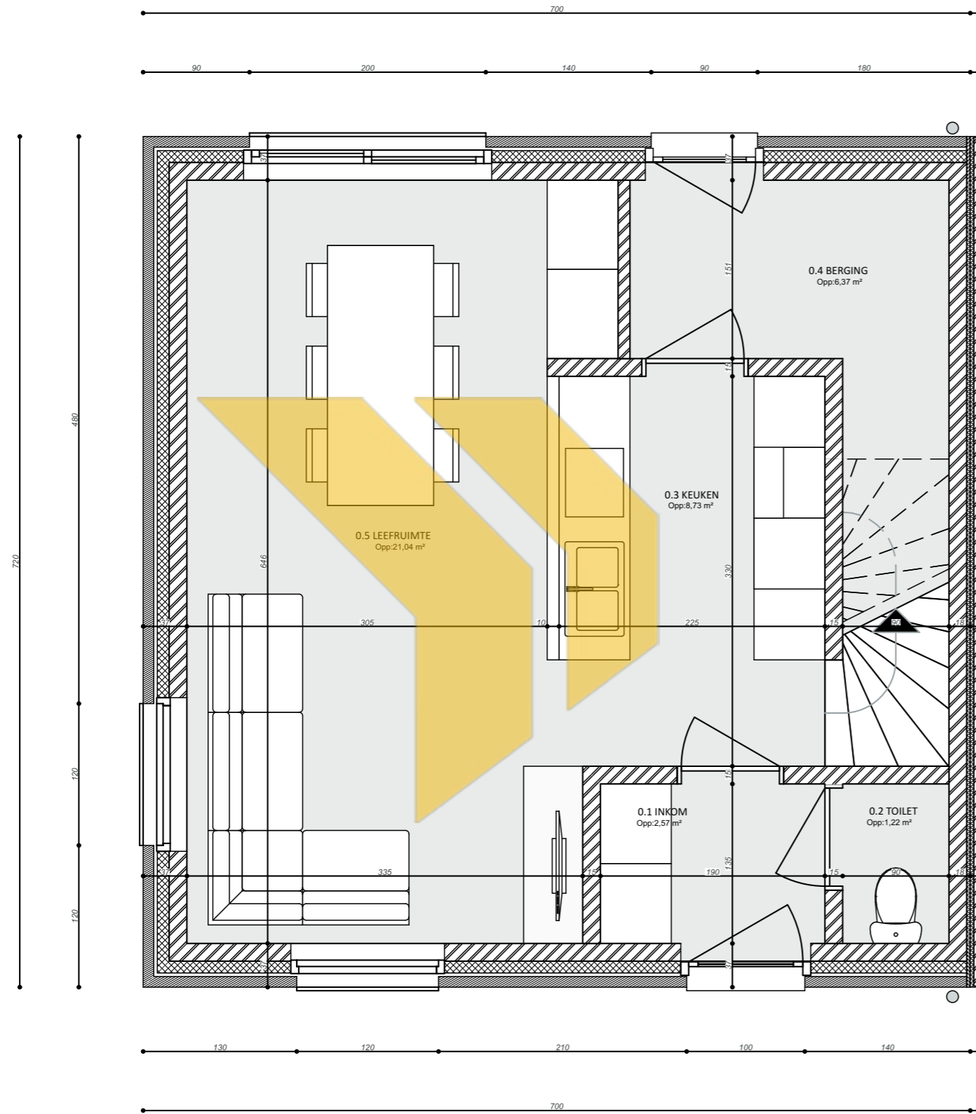
MHOB1/H GELIJKVLOERS A: 50,40 m 2
