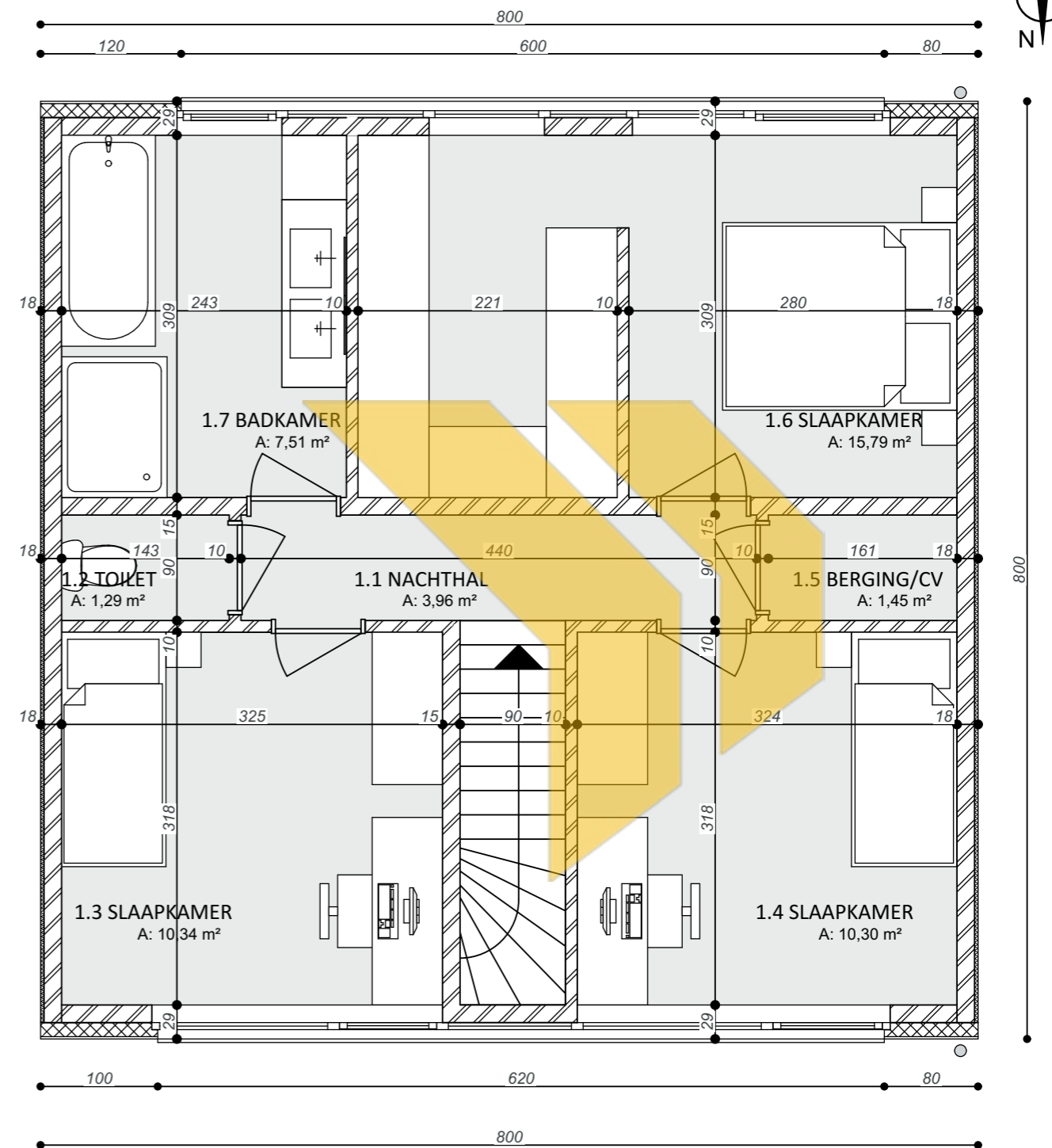
MGB 3/P VERDIEPING A: 64,00 m²
