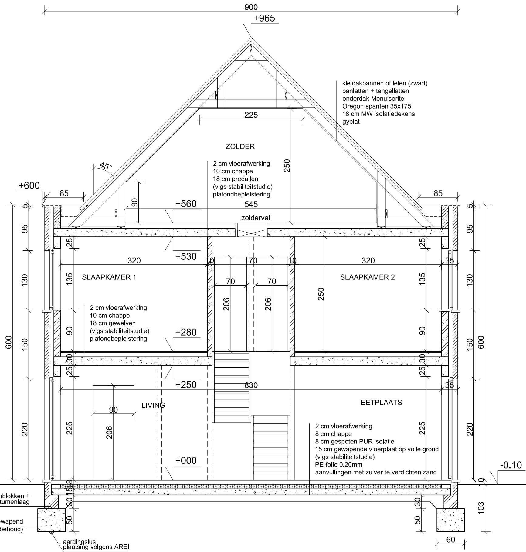
TYPEDOORSNEDE
