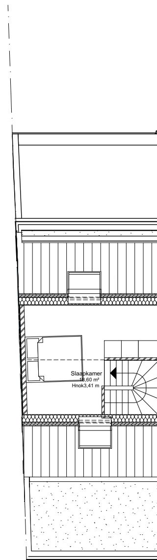
2. Lot 1 - 2e verdieping 1:100
