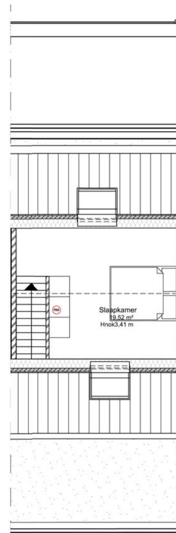
2. Lot 5 - 2e verdieping 1:100
