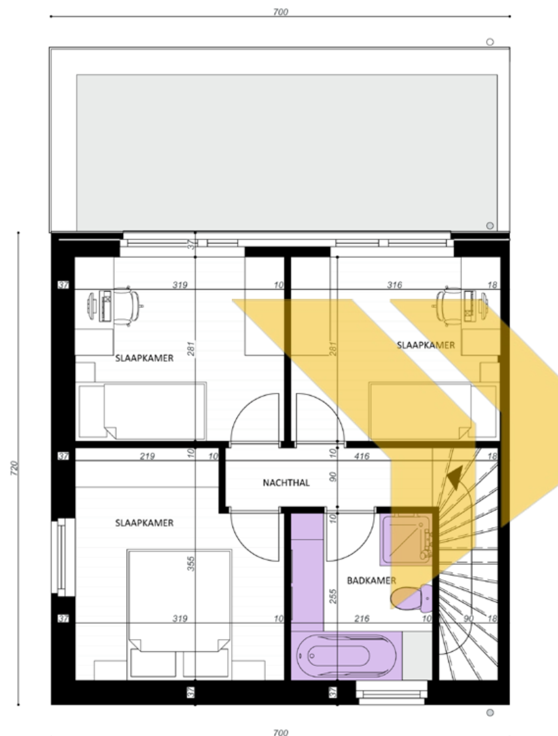
MHOB 7 - Verdieping A: 50,40 m 2
